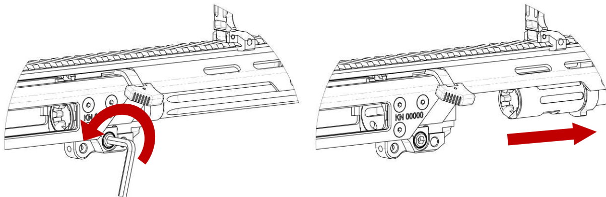
Rys. 34. Demontaż lufy
