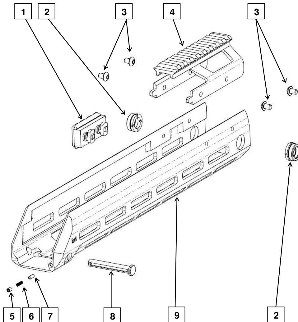
Rys. 22. Zespół łoża przedłużonego M-LOK: 1 – zespół szyny (3 sloty); 2 – gniazdo pasa; 3 – wkręt mocujący nakładkę; 4 – nakładka łoża; 5 – wkręt dociskowy M3; 6 – sprężyna zawleczonego łoża i komory spustowej; 7 – kołek blokujący; 8 – łącznik łoża; 9 – łożo wersja A2
