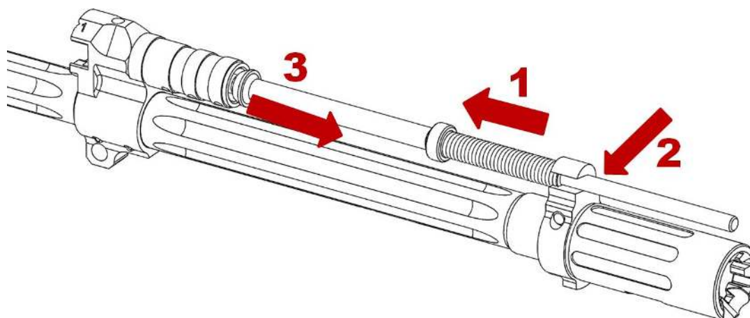
Rys. 35. Rozłożenie lufy
