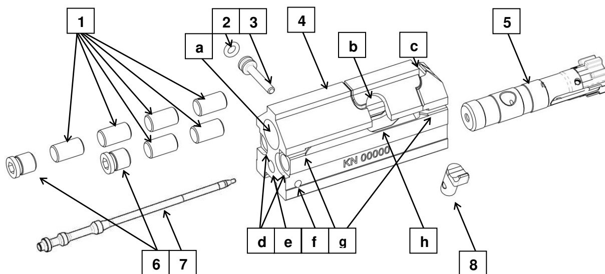
Rys. 11. Suwadło z zamkiem: 1 – bezładniki; 2 – pierścień gumowy; 3 – kołek iglicy; 4 – suwadło; 5 – zespół zamka; 6 – śruby zabezpieczające urządzenia przeciwostrzałowego (wkrętki suwadła); 7 – iglica; 8 – trzpień sterujący zamka (wodzik); a – gniazdo sprężyny powrotnej; b – wycięcie do demontażu trzpienia sterującego zamka; c – wybranie współpracujące z zębem tylnym zapadki napinacza; d – gniazda bezładników; e – gniazdo iglicy; f – gniazdo kołka iglicy; g – wycięcie prowadzące suwadła; h – krzywka suwadła
